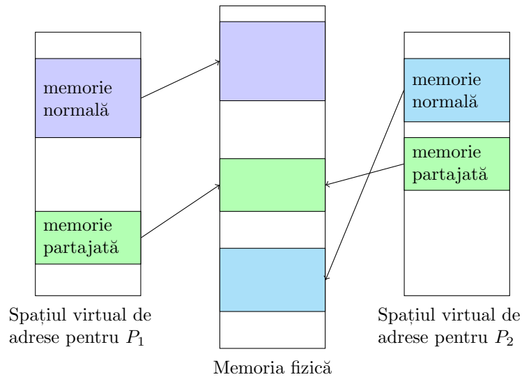
Figura 12.1: Modul în care sistemul de operare implementează conceptul de memorie partajată
