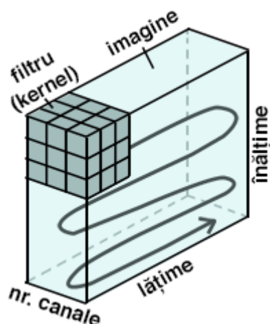
Figura 4. Deplasarea unui kernel într-o imagine în timpul operației de convoluție.
