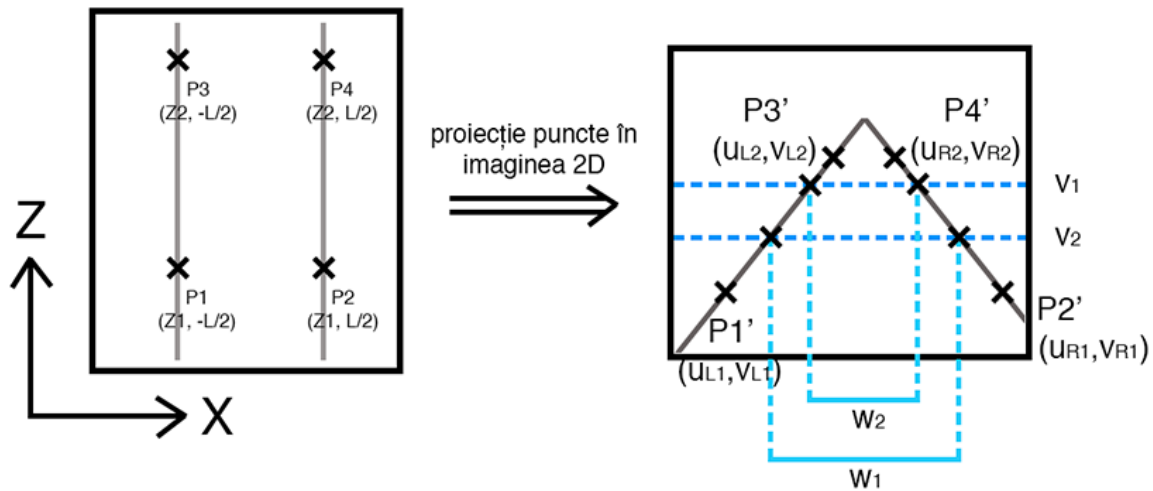
Figura 93. Determinarea celor două lăţimi w_1 şi w_2 .
