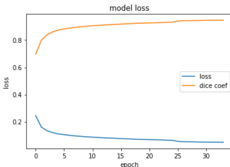
Figura 27. Rezultatul antrenării după 34 de epoci: funcția de cost ("loss") scade, iar coeficientul Sorensen-Dice ("dice coeff") converge spre valoarea 1.
