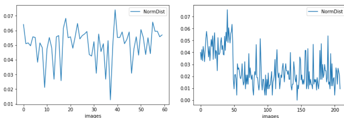
Figura 80. NormDist calculat pe baza de date de validare: 59 imagini din oraș (sus) și 209 imagini de pe autostradă (jos).
