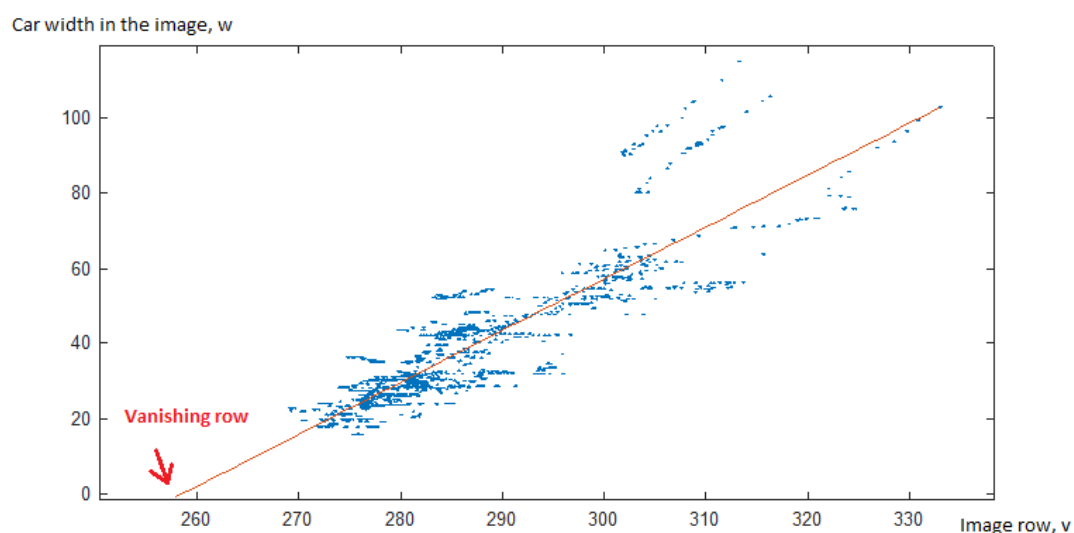
Figura 94. Relația liniară între lățimea unei mașini și coordonata de jos a chenarului de încadrare a vehiculului pe axa orizontală (coordanata linei).
