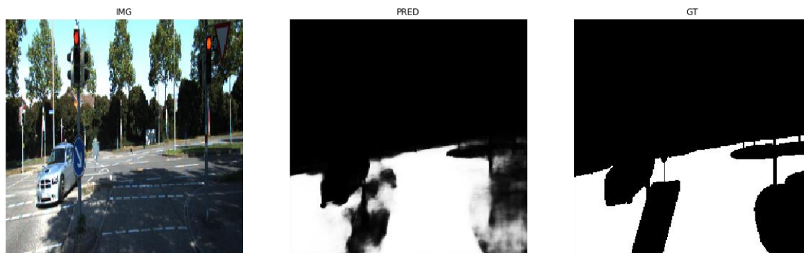
Figura 34. Rețeaua are anumite dificultăți în zone de umbră și iluminare neuniformă a scenei. Sursă imagini: [Geiger2012].
